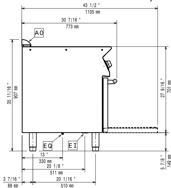
Zij aanzicht
